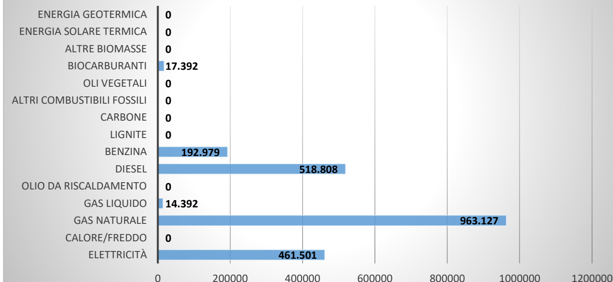
Grafico 38 Consumo energetico finale per vettore nell'anno di riferimento 2010
